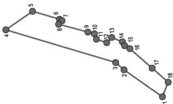
Чертеж и каталог координат 70:22:0010109:ЗУ 7
