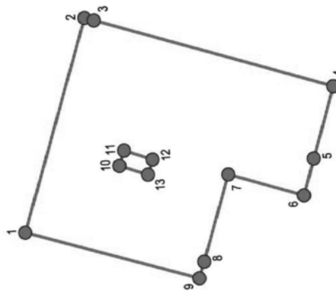
Чертеж и каталог координат 70:22:0010109:3У 2
