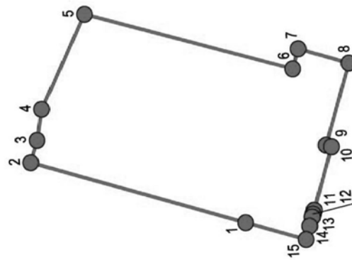
Чертеж и каталог координат 70:22:0010109:3У 1
